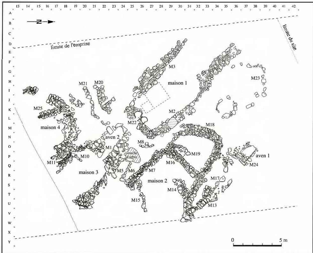
Figure 3 : Le site Néolithique final des Vauts (Saint-Gély-du-Fesc, Hérault). Plan des unités d'habitation en pierre sèche (D'après Guilaïne, Escallon, 2003. DAO : A. Burens-Carozza, Collège de France).
