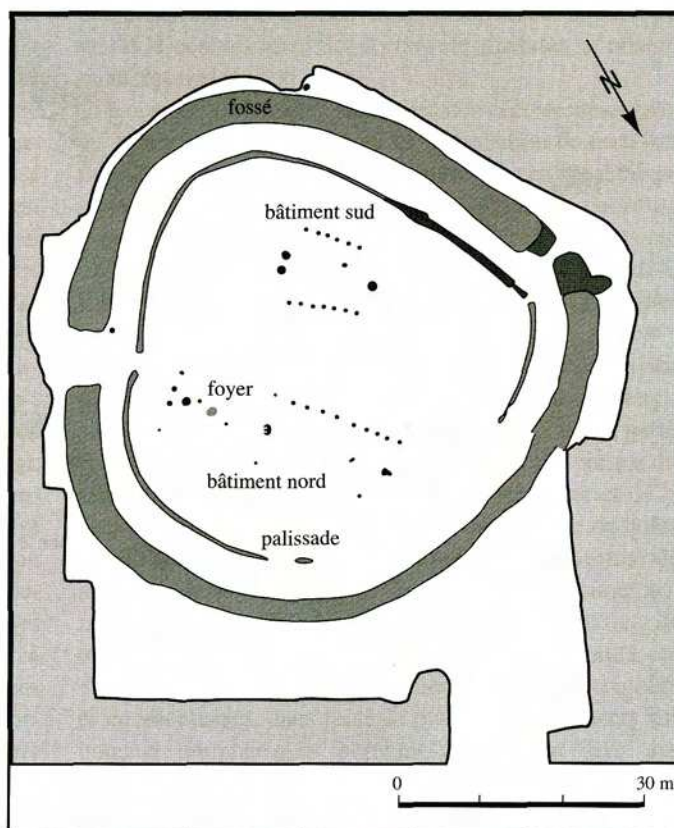
Figure 4 : Le Mourral, Trèbes (Aude). Plan du site d'après les données de la fouille. Les zones plus sombres de la palissade et du fossé correspondent à des zones recreusées au cours de l'occupation ancienne du site (Relevé J. Vaquer).
